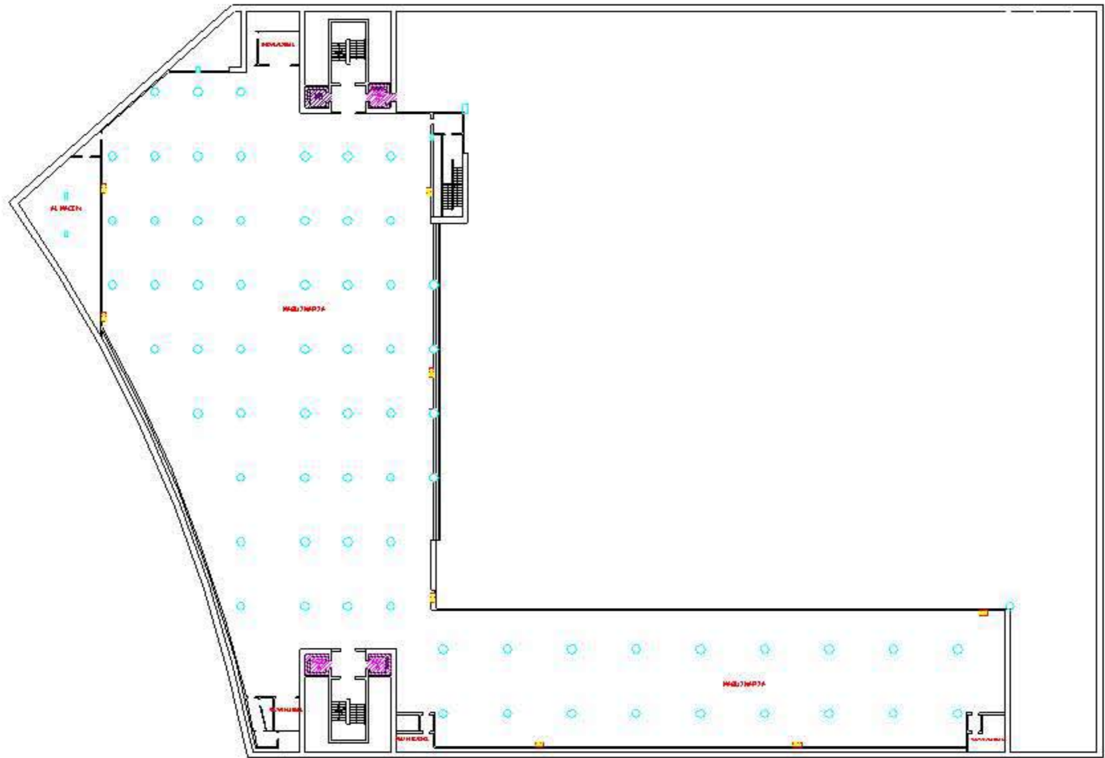
PLANTA -7 (COTA -17.97)
